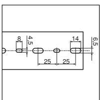
Götun botns Samkvæmt EN 50085 á rennum sem hafa 25/40/60 mm breidd
