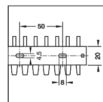
Götun í botni VK flex 40
