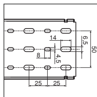
Götun botns Samkvæmt EN 50085 á rennum sem hafa 80/100/120 mm breidd
