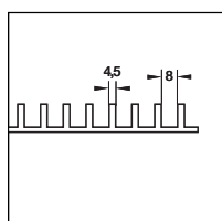
Hliðarmál VK flex 10
