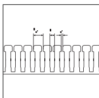
Hliðarmál Rennur sem hafa 25/40 mm hæð
