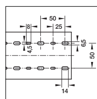
Götun í botni samkvæmt DIN 43659. Rennubreiddir 75, 100 og 125 mm
