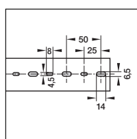
Götun í botni samkvæmt DIN 43659. Rennubreiddir 25, 37, 50 mm
