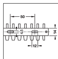
Götun í botni VK flex 20 og 30
